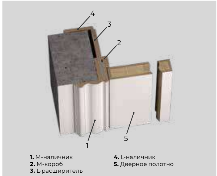
Обратное открывание
