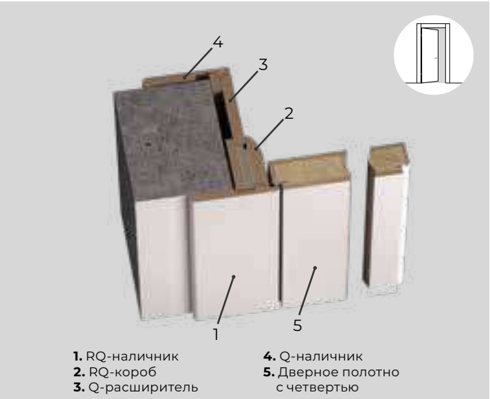
Обратное открывание
