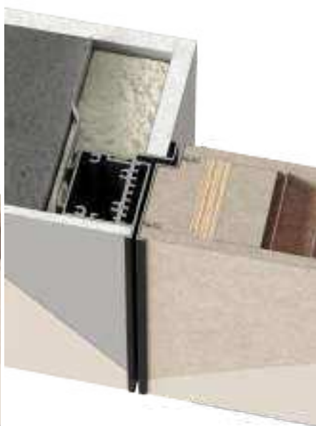
Ultimatum Схема-разрез прямого открывания для дверного полотна 59 мм
