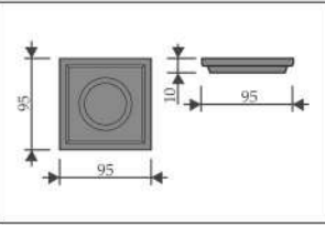
ПРИТВОРНАЯ ПЛАНКА
