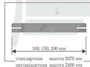
ДОБОРНАЯ ПЛАНКА №2/2
