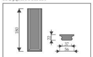
ПОДПЯТНИК
