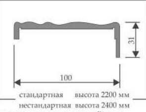
КАРНИЗ СБОРНЫЙ №4
