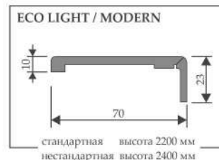
ПРИТВОРНАЯ ПЛАНКА
