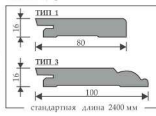
ПЛИНТУС
