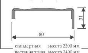
ПОДПЯТНИК
