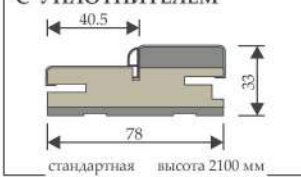
ДОБОР №2/2
