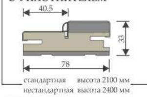
САНДРИК №4
