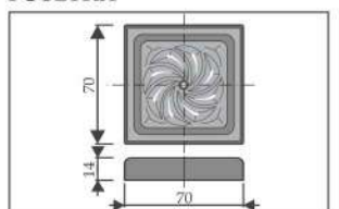
РОЗЕТКА
