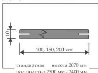
ДОБОРНАЯ ПЛАНКА
