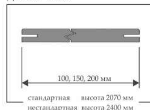
ДОБОР №2/2
