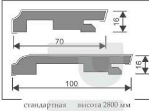
ПЛИНТУС НАПОЛЬНЫЙ
