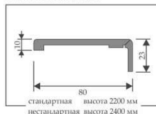
ПРИТВОРНАЯ ПЛАНКА
