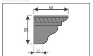
КАРНИЗ
